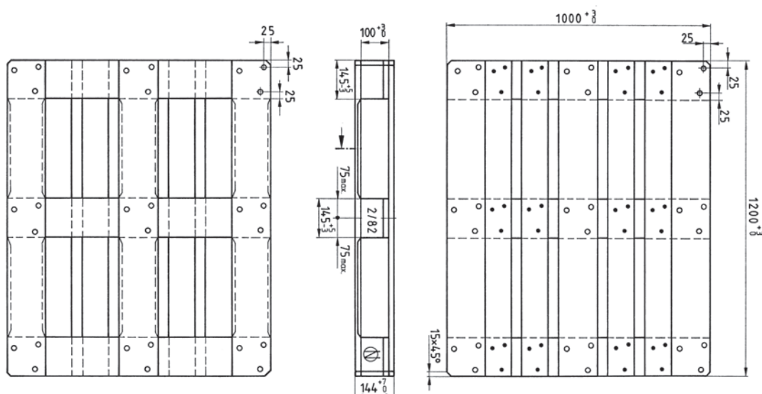
Europalette EUR3
